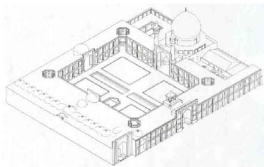
تصویر ۱- نمای سه‌بعدی مدرسه چهارباغ (حاجی قاسمی، ۱۳۷۹: ۴۶).
